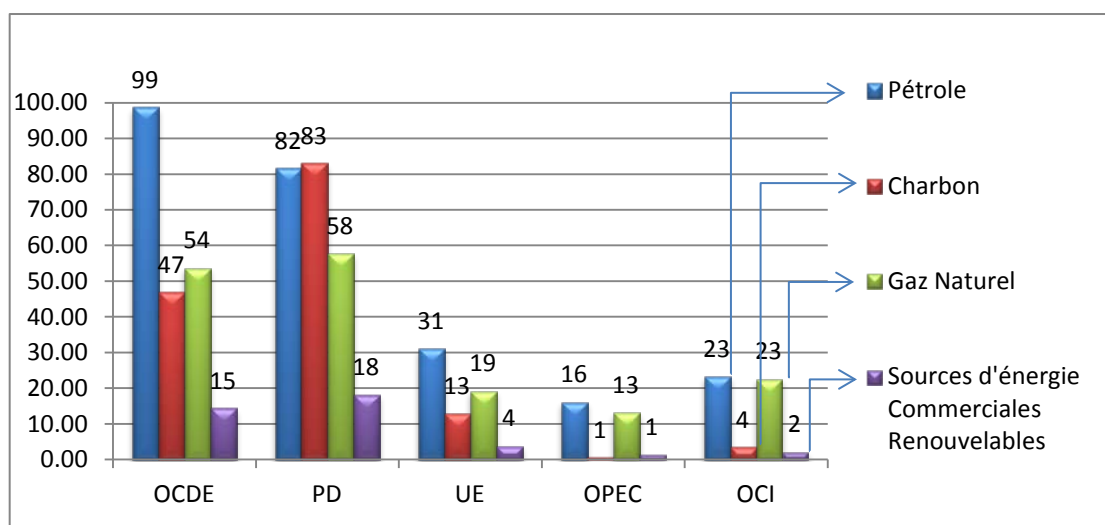
Schéma 8 : Consommation des Sources d'Énergie Commerciales dans des Pays de l'OCI et d'Autres Régions (Quadrillion UTB), 2006
