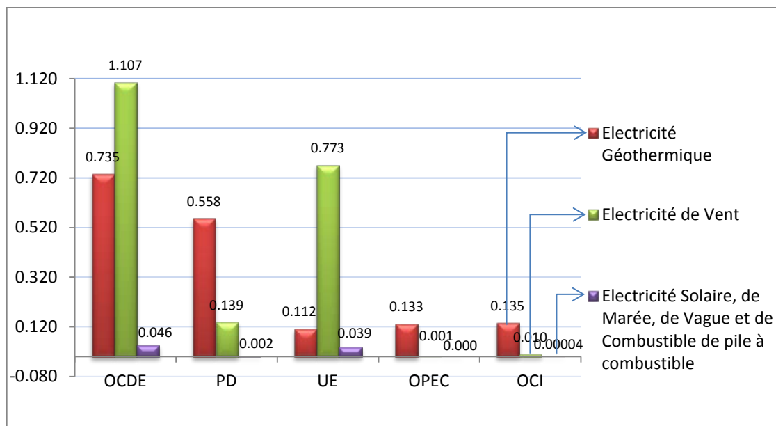
Schéma 10 : Consommation Nette des Sources Renouvelables Non-Hydro-électriques de l'Électricité dans les Pays de l'OCI et d'Autres Régions (Quadrillion UTB), 2006
