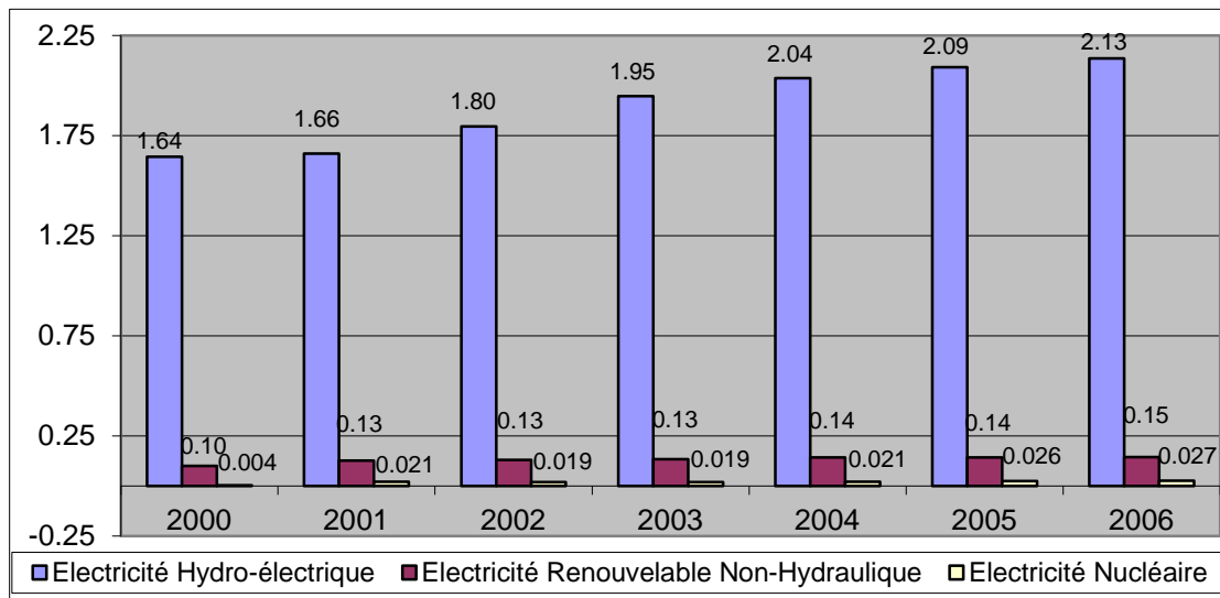
Schéma 5 : Consommation Nette de l'Électricité Renouvelable de Courant, Hydro-électrique et Non-Hydro-électrique Électrique Nucléaire dans des Pays de l'OCI (Quadrillion UTB), 2000-2006
