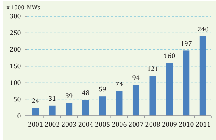
الشكل 4.6: إجمالي طاقة الرياح المثبتة في العالم (ألف ميغاوات)
