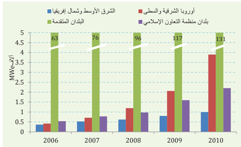
الشكل 5.6: مجموع منشآت الرياح حسب الأقاليم (ألف ميغاواط)
